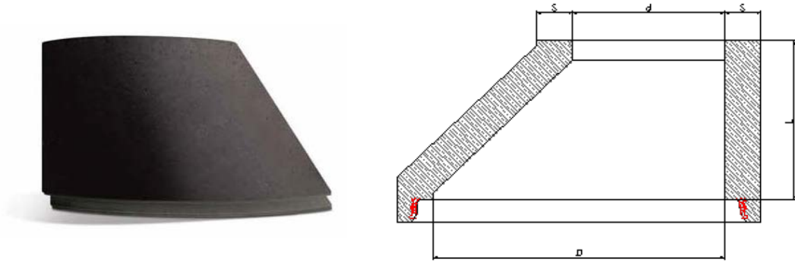
Şekil 1.4. Baca konisi
