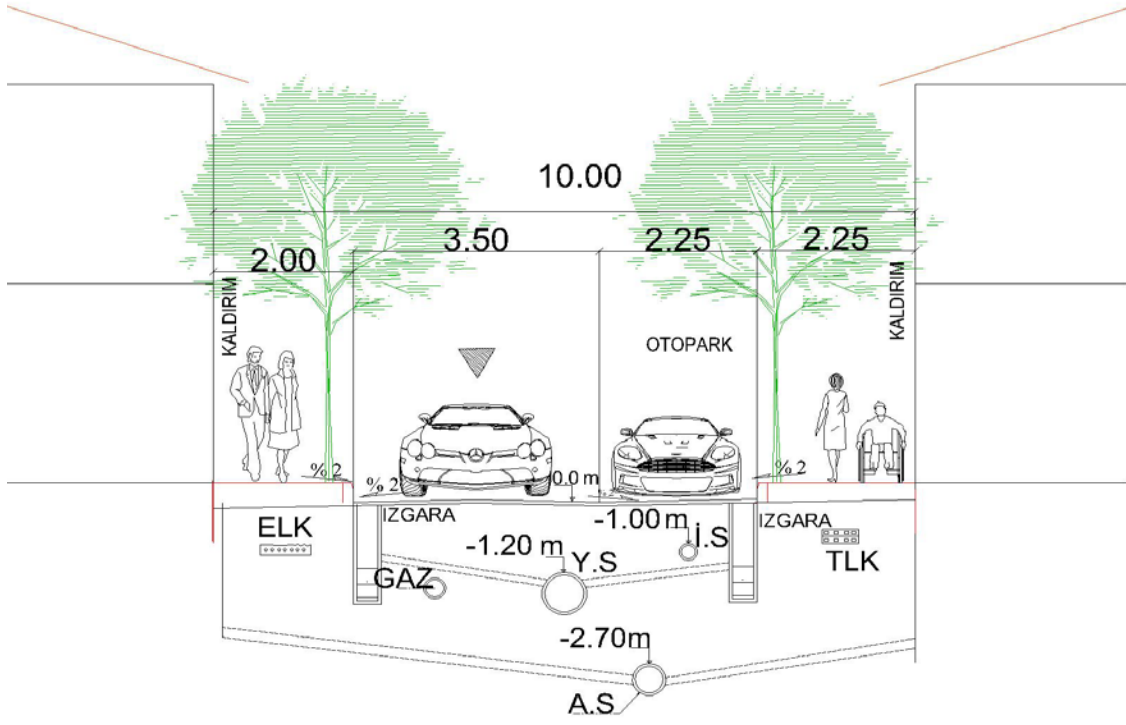
Şekil 1.13. 10 m’lik servis veya yaya yolu için teknik altyapı sistemlerinin konumlandırılması Seçenek-II
